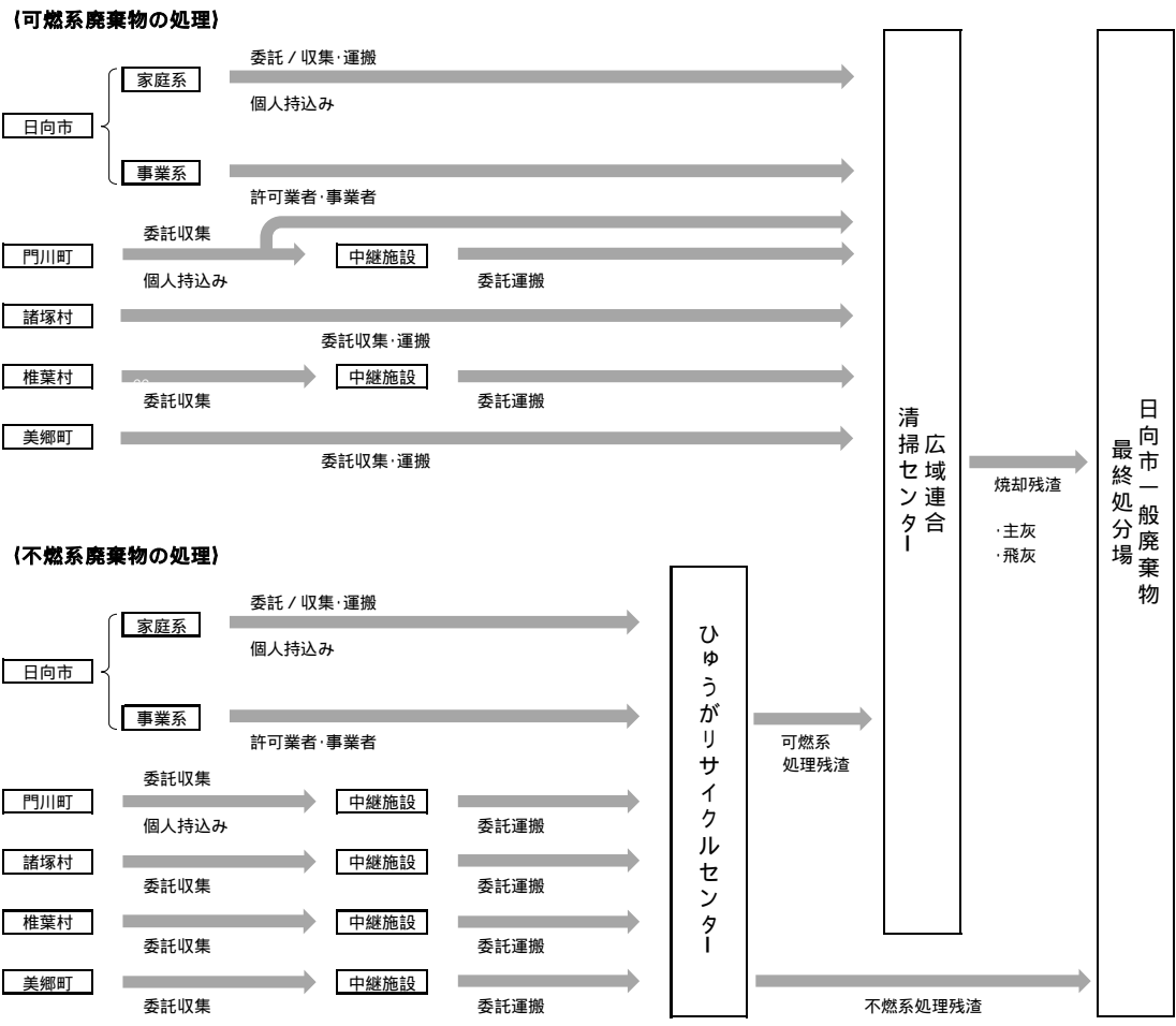
図 2 ごみ処理体制
