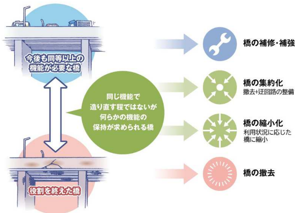
図 23 道路橋の集約・撤去方針
