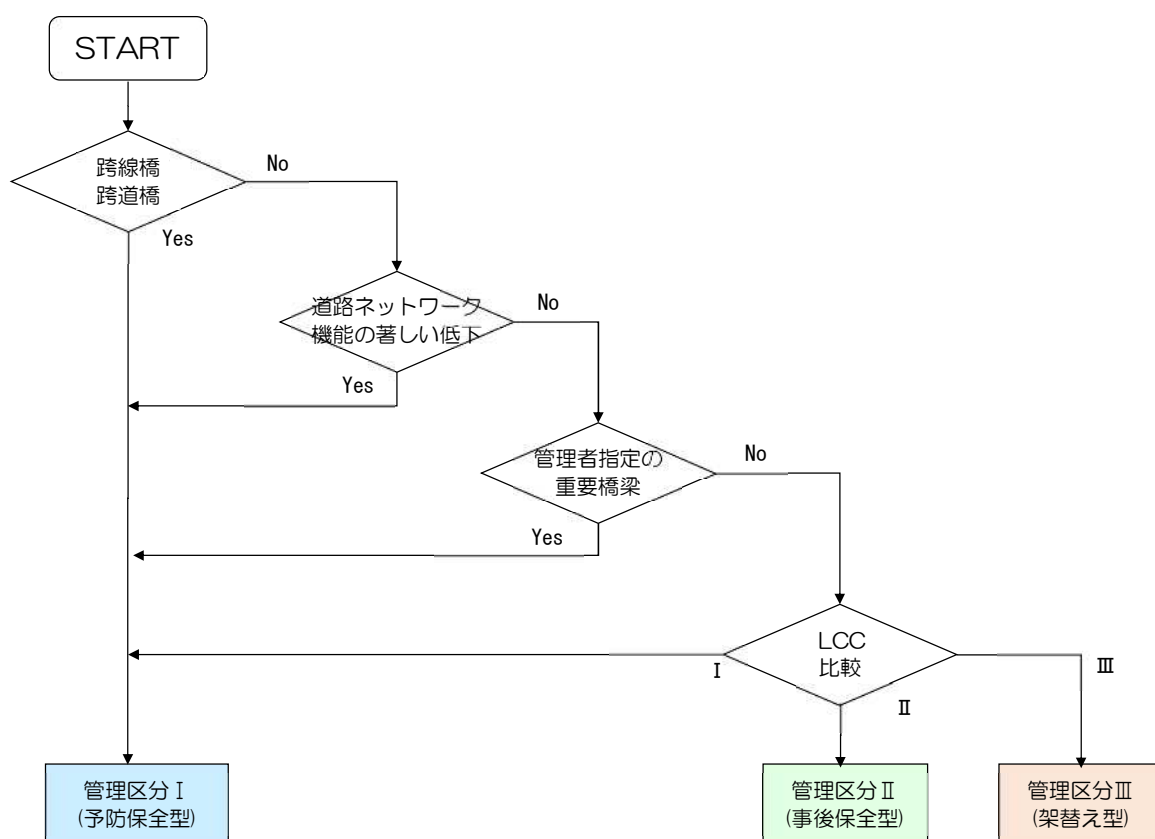
図 14 橋梁ごとの維持管理方針の最適化
